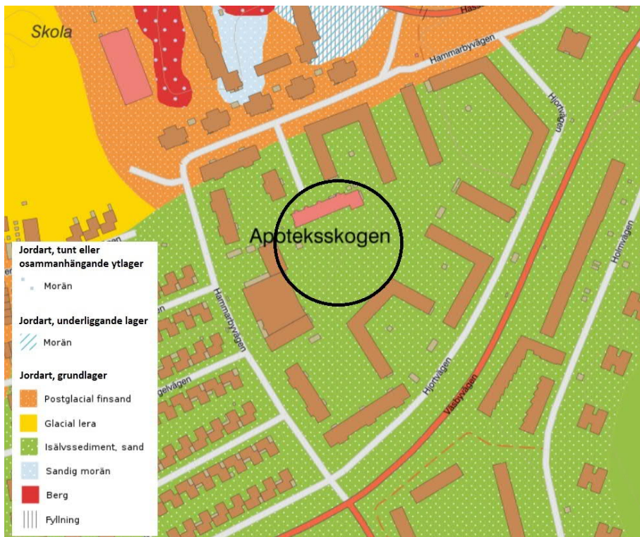
Figur 2. Utklipp från SGU:s jordartskarta (SGU, u.å.a). Ungefärligt undersökningsområde är markerat med svart cirkel.
