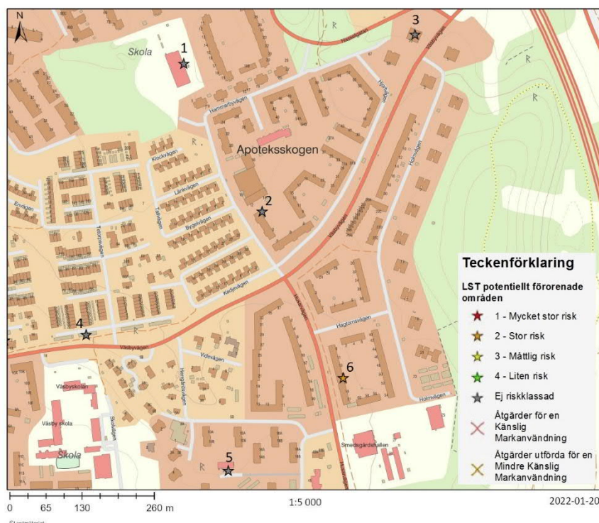
Figur 6. Karta över de sex potentiellt förorenade områden inom och i närheten av undersökningsområdet. Källa: Vatteninformationssystem Sverige 2022-01-20 (VISS, u.å.).
