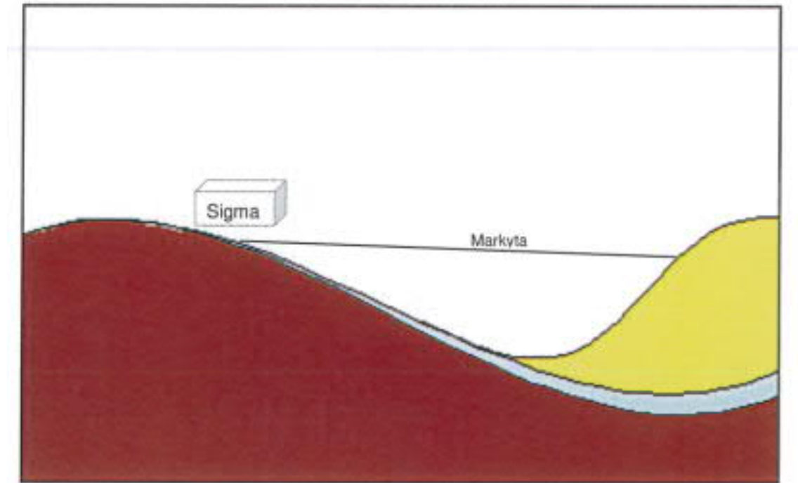
Figur 3. Urklipp från Sweco:s Hydrogeologisk rapport, Sigma, Upplands Väsby. Daterad 2010-04-20 (Sweco, 2010a). Undersökningsområdet markeras med rött.
