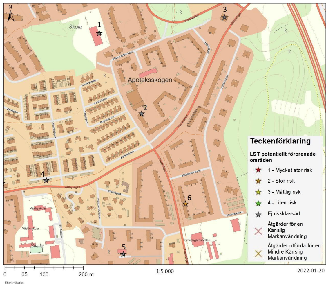
Figur 5. Karta över de sex potentiellt förorenade områden inom och i närheten av undersökningsområdet. Källa: Vatteninformationssystem Sverige (VISS), 2022-01-20.
