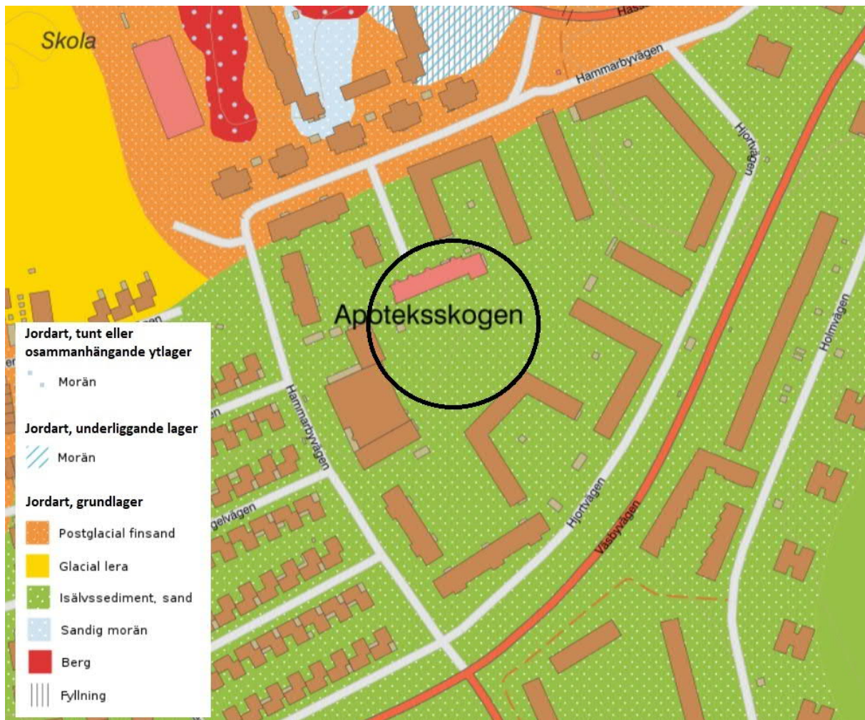
Figur 2. Utlägg från SGU:s jordartskarta (SGU, u.å.a). Ungefärligt undersökningsområde är markerat med svart cirkel.
